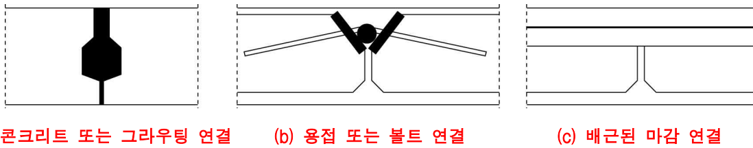
그림 4.7-2 전단력 전달을 위한 연결부의 예
