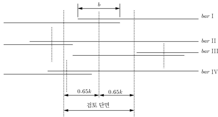
그림 4.5-11 하나의 단면에서 겹침이음된 철근의 비율
