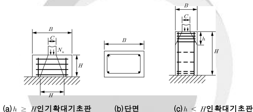
그림 4.6-15 암반 위 기둥의 쏄임 방지 철근
