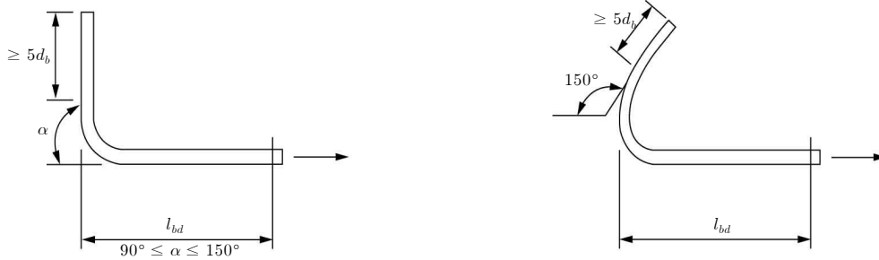
(a) 구부림 각도가 90°에서 150° 사이인 갈고리 (b) 구부림 각도가 150° 이상인 갈고리
